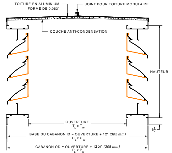
COINS À ONGLET *OPTIONNEL PH-2625M
